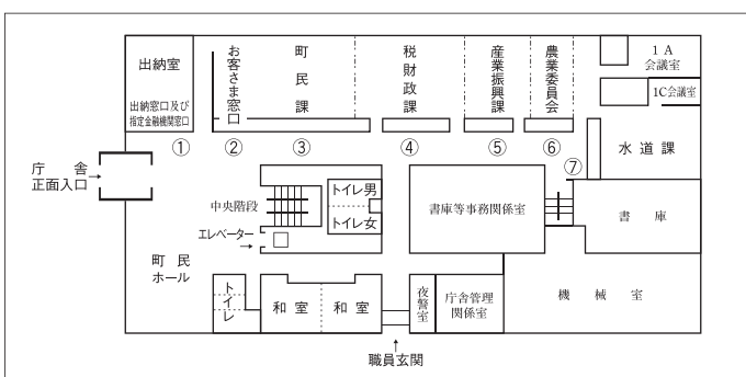
■庁舎1階平面図
