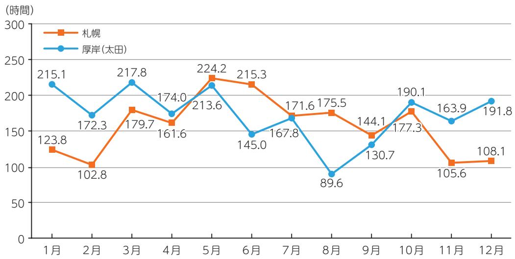
月別日照時間(令和5年)
