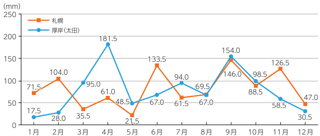
月別降水量(令和5年)
