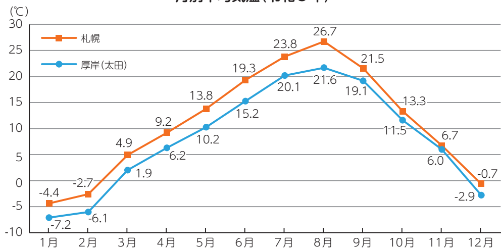
月別平均気温(令和5年)
