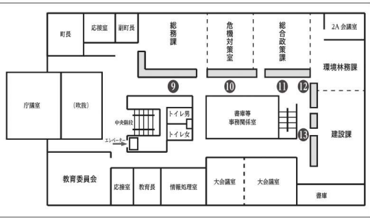
■庁舎2階平面図
